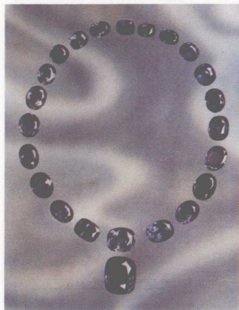
19、蓝宝石戒面
