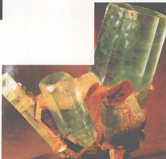
26、绿柱石晶体
