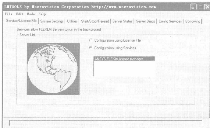
图 1.12 LMTOOLS 窗口 1
