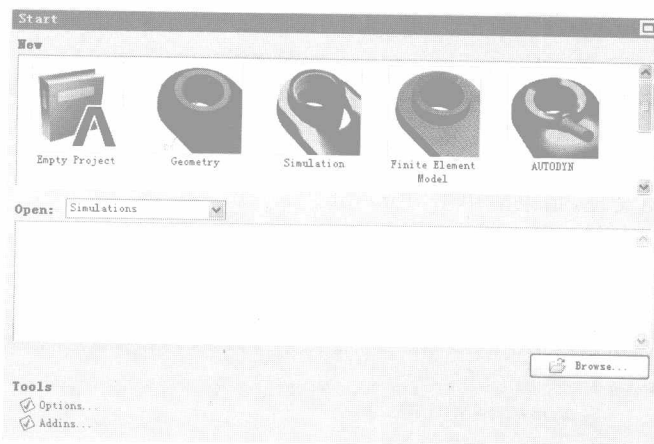
图 1.14 Start 窗口
