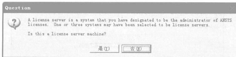
图 1.9 Question 窗口 1
