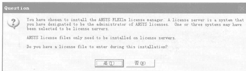
图 1.10 Question 窗口 2
