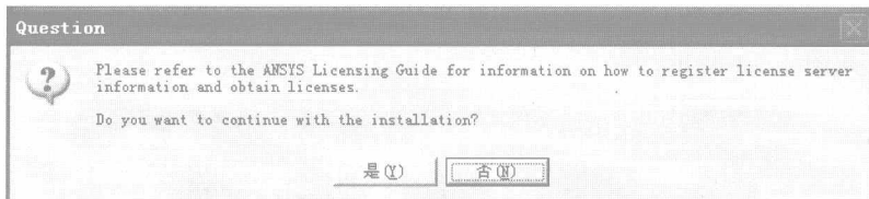
图 1.11 Question 窗口 3
