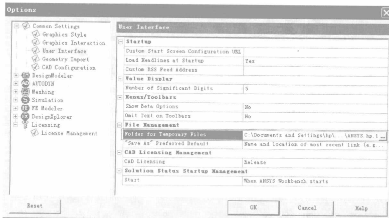
图 1.15 Options 窗口
