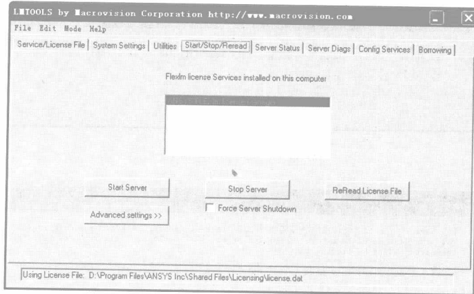
图 1.13 LMTTOOLS 窗口 2
