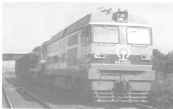
1989年3月22日，大连机车车辆工厂与美国GE公司合作，研制成功第一台东风6型内燃机车
