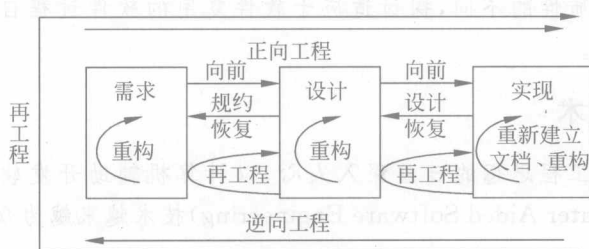
图 2 软件再工程
