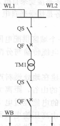
图 1-4 支接变电所示意图
