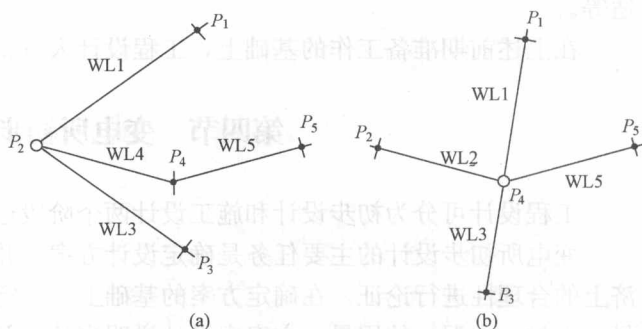
图 1-8 变电所位置的确定方案比较
