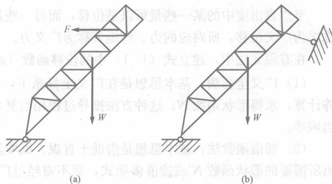
图 1-1 井架起升工况时的力学模型
