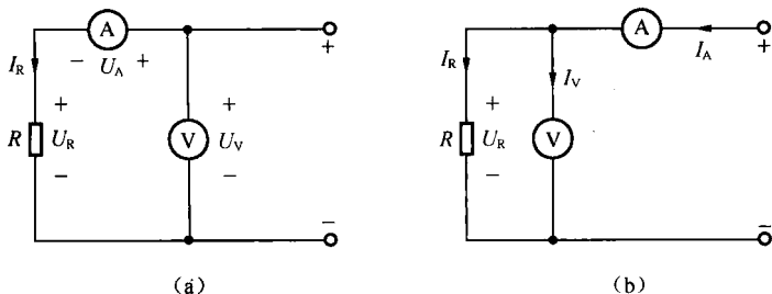
图 1-1-2 间接法测量电阻
