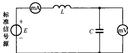
图 1-1-3 测量电感或电容
