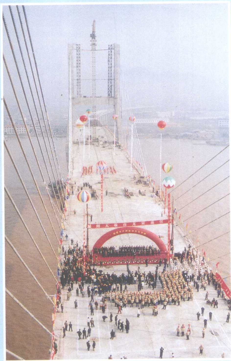
1997年12月16日，温州大桥胜利合龙，该桥全长17.1公里，总投资11.79亿元，是目前我国最长的公路大桥 张环清 摄
