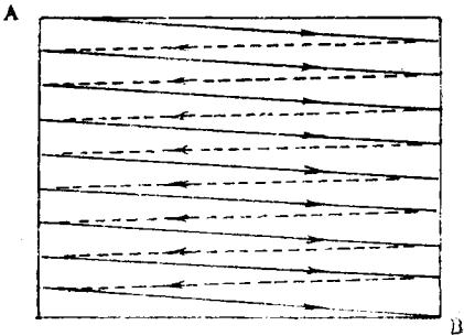
图 1—4 逐行扫描示意图
