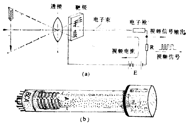
图 1—3 摄象管结构示意图
