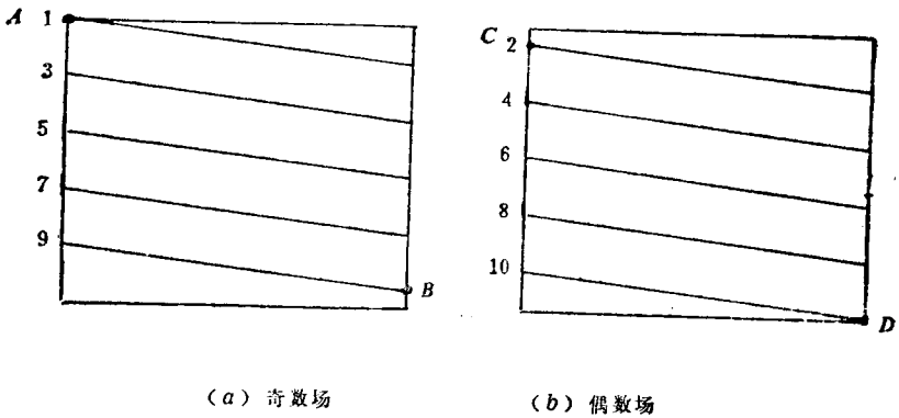
图 1—7 总行数为偶数的隔行扫描
