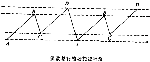
偶数总行的场扫描电流
