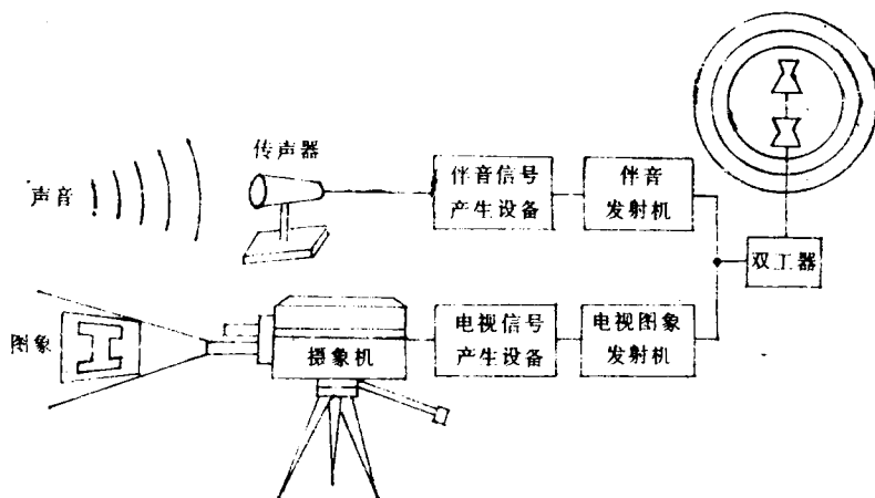
图 1—1 电视发送示意图
