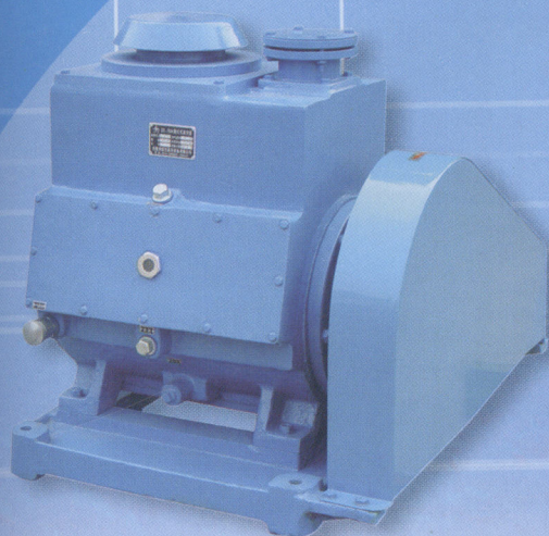
↑ 2X 型旋片式真空泵
