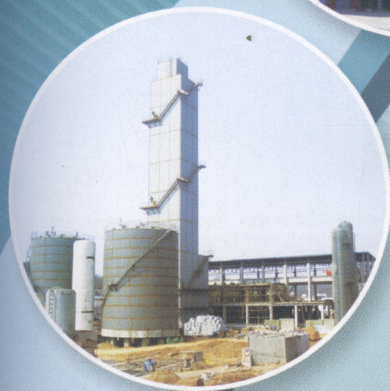
↑ 为南阳汉冶提供的 KDON (Ar)-20000/20000/700 型空分设备
