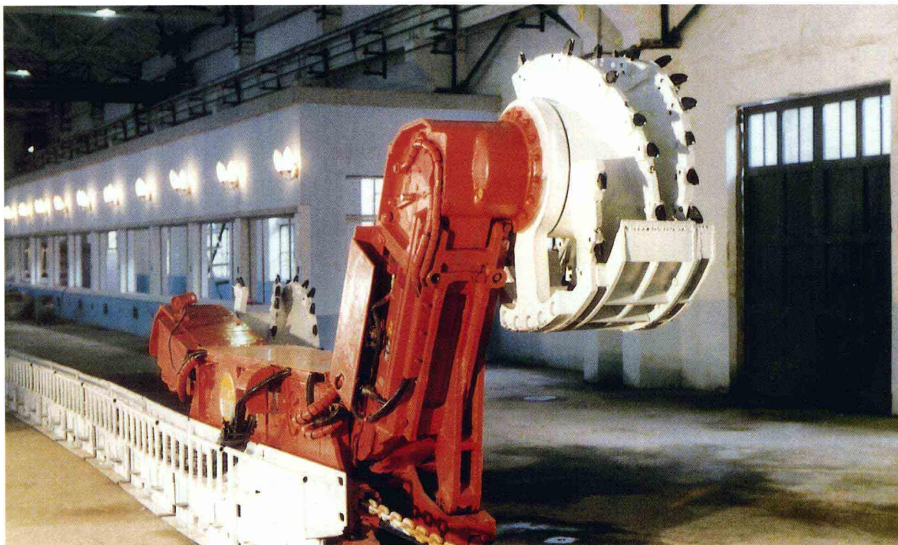
西安煤矿机械厂生产的采煤机
