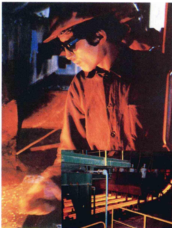
中国第一套30吨电弧炉R5.25方坯连铸机 在西安钢铁厂建成
