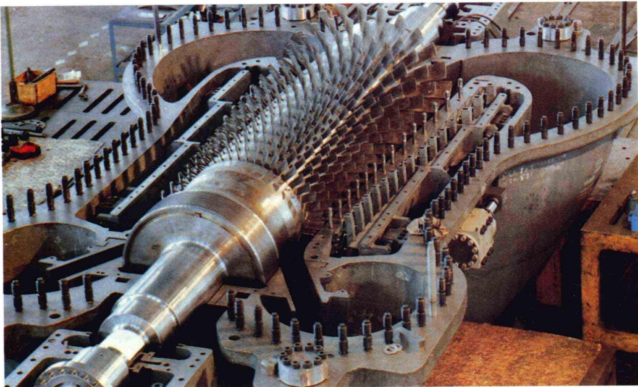
陕西鼓风机厂研制生产的轴流压缩机剖面
