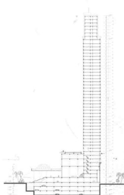
酒店立面图
