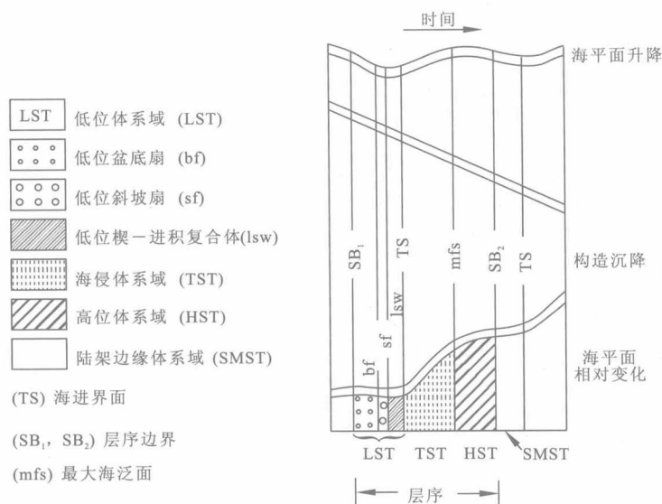
图 1-1 海平面变化与体系域关系
