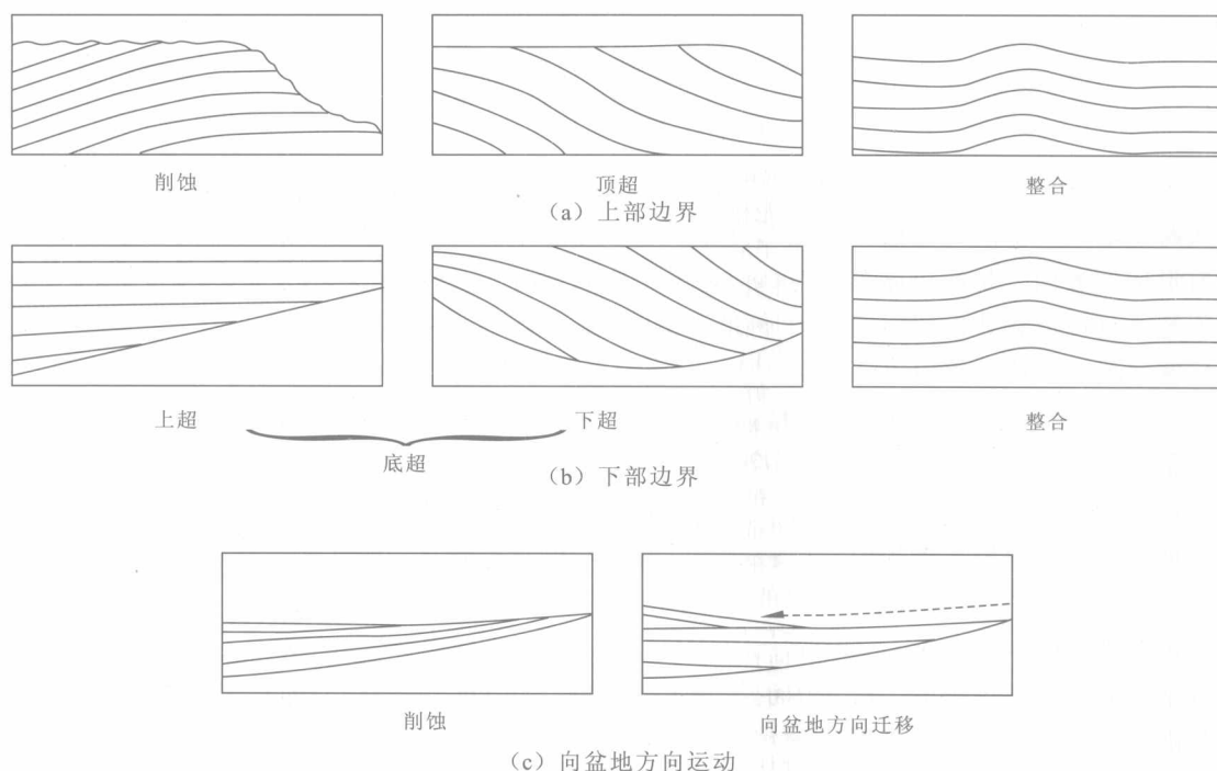
图 1-3 地层与层序边界之间的关系示意图
