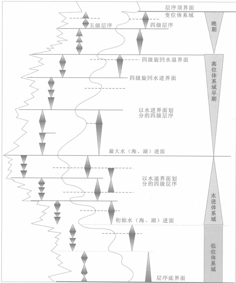
图 1-2 一个三级层序内的四级和五级高频层序单元划分 (据林畅松，2002)
