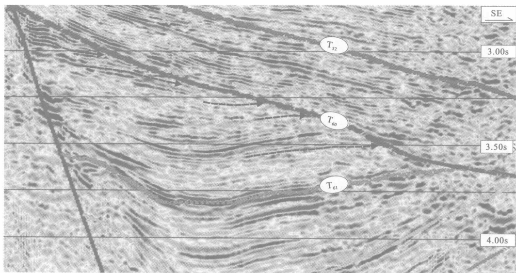
图 1-4 琼东南盆地 97D1023 测线示 T_{60} 界面，一个不整合层序边界与其他层序边界之间的接触关系 (据王华等，2005)
