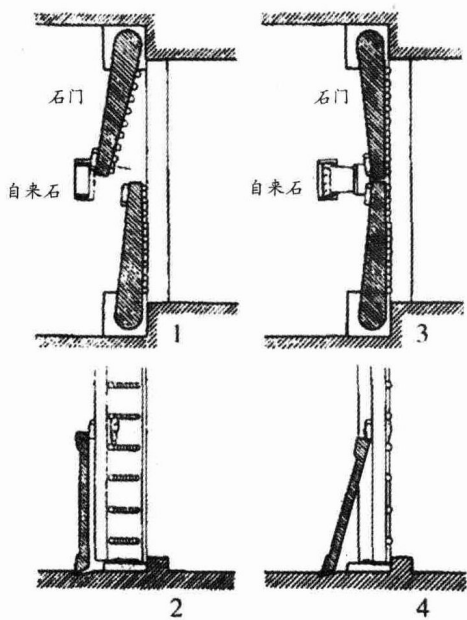
地宫石门关闭示意图 1.关闭前 (平面) 2.关闭前 (侧面) 3.关闭后 (平面) 4.关闭后 (侧面)
