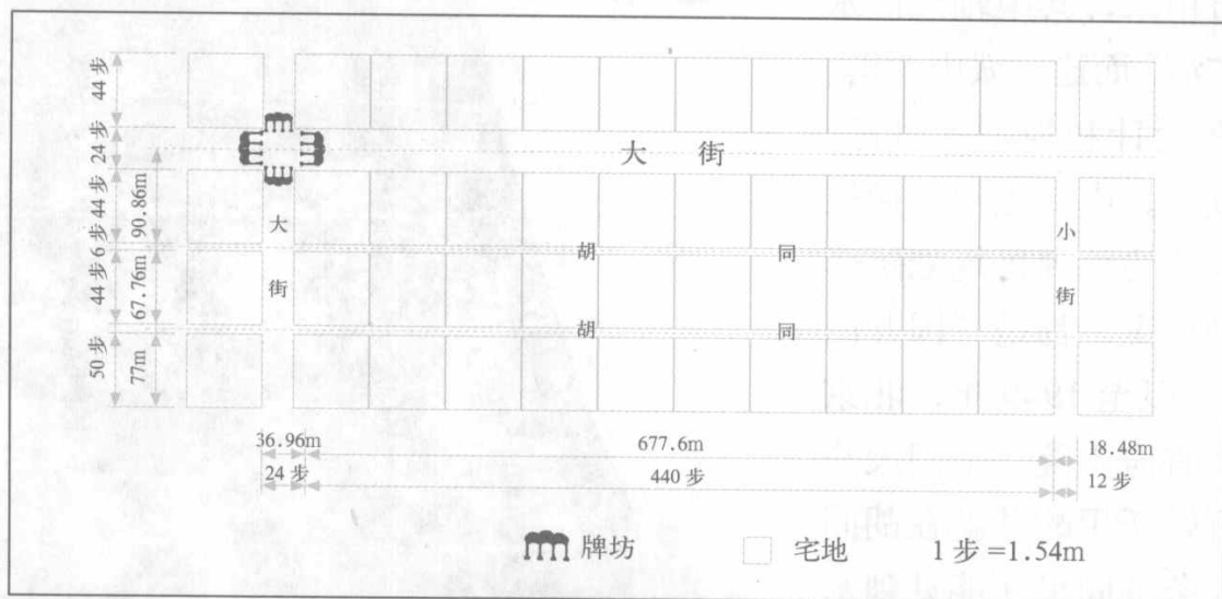
● 图 1-6 元大都街区构成模式图
