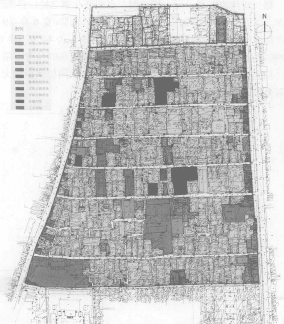
● 图1-5 西四北头条—八条平面示意图
