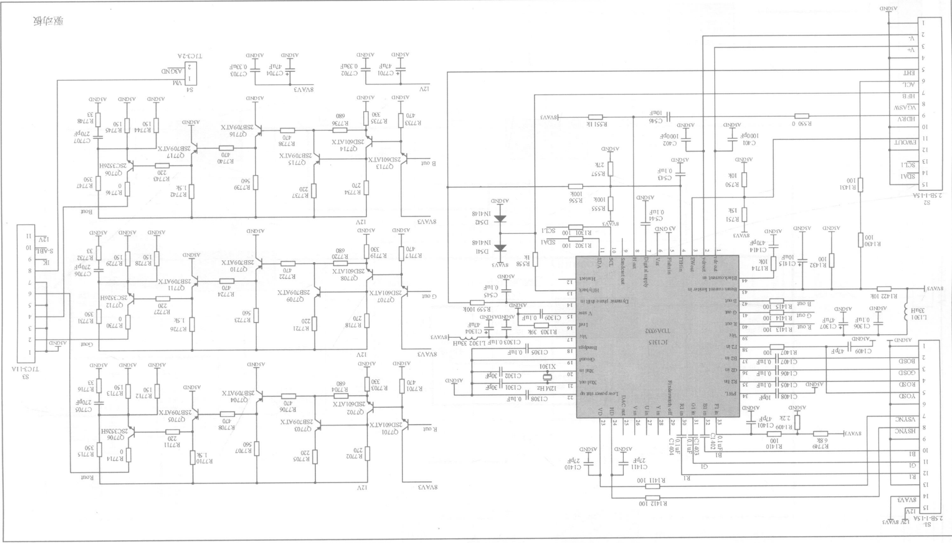
43PTV 机芯彩色电视机电路原理图 (5/13)
