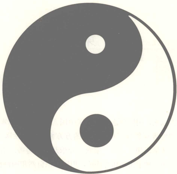
图 1-2 阴阳太极图
