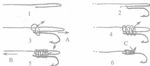
图 5 怎样拴钩
