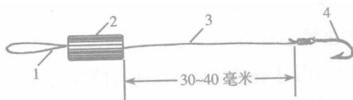
图 7 引线长度
