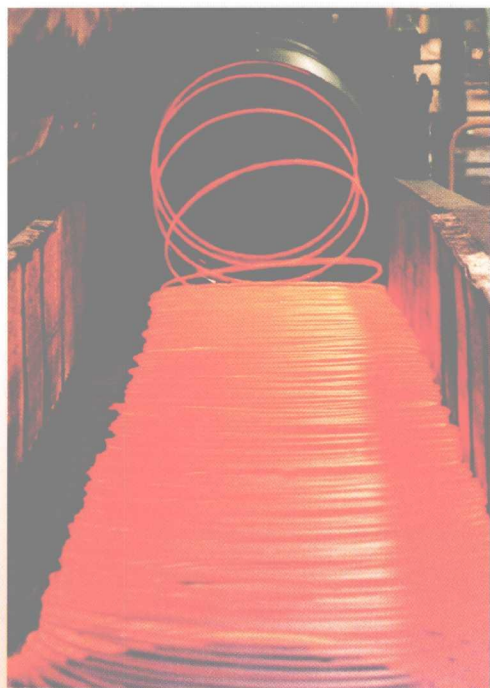
大钢集团棒线材连轧机吐丝
