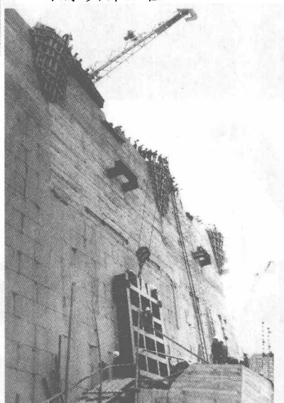
技术人员在进行落闸试验 取水头部工程
