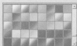
渐变
