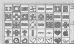
形状
