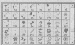
画笔
