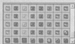
样式
