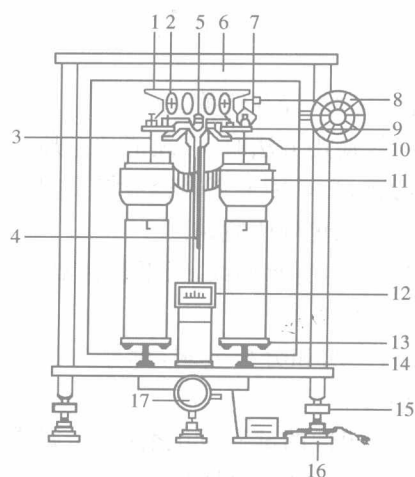
图 1-1 电光分析天平示意图
