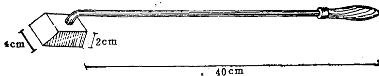
图 4-7 方形烙铁
