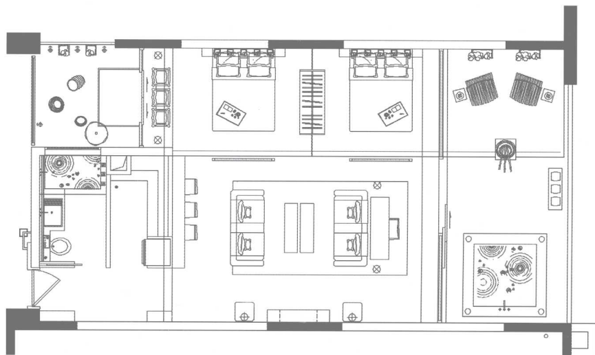
平面布置图
