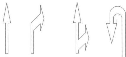
㉕ 计算行车速度 \leq 40\text{km/h} 时的导向箭头
