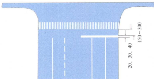
④⑥ 停止线 (尺寸cm)。是与道路中心线相垂直的一条白色实线,表示车辆等候放行信号或停车让行时的停车位置。
