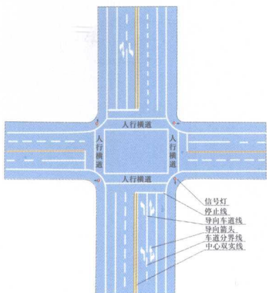
④⑤ 信号灯路口的停止线
