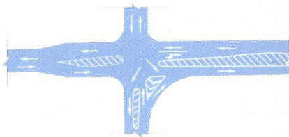
④⑫ 复杂行驶条件十字路口导流线
