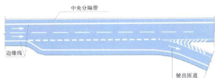
⑯ 平行式出口标线
