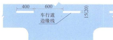
⑥ 边缘线的尺寸(cm)
