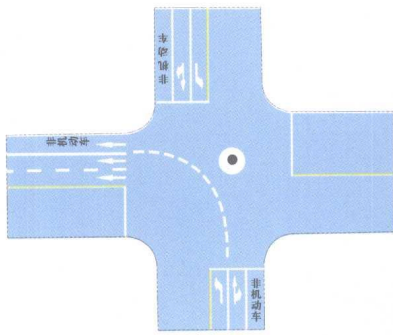
⑧ 左转弯导向线
