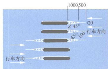
㉔ 收费岛地面标线
