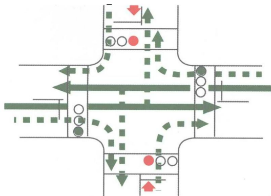
① 红绿灯指挥信号
