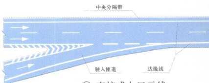
⑰ 直接式入口示线
