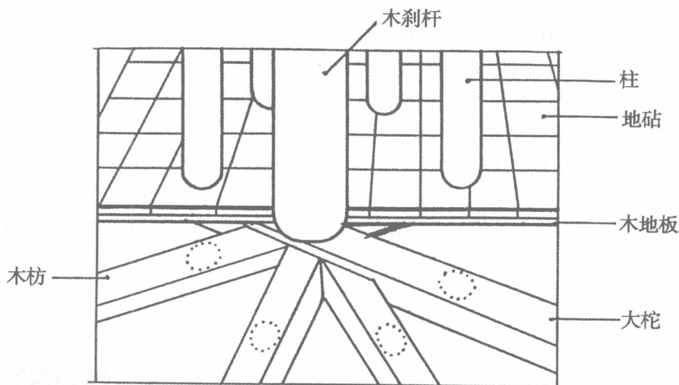
刹木底部透剖图
