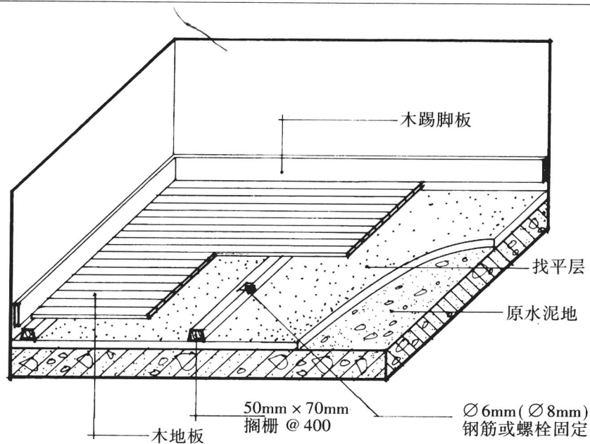
图 10 单层架空木地板构造图
