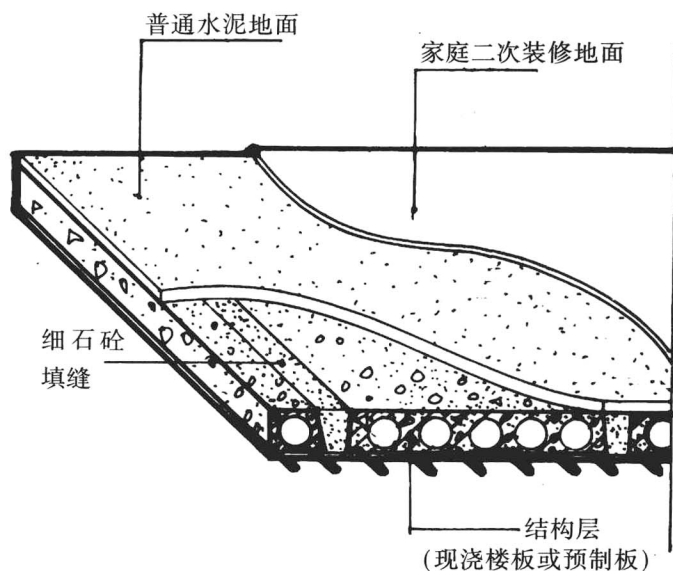
图3 楼层地面构造图
