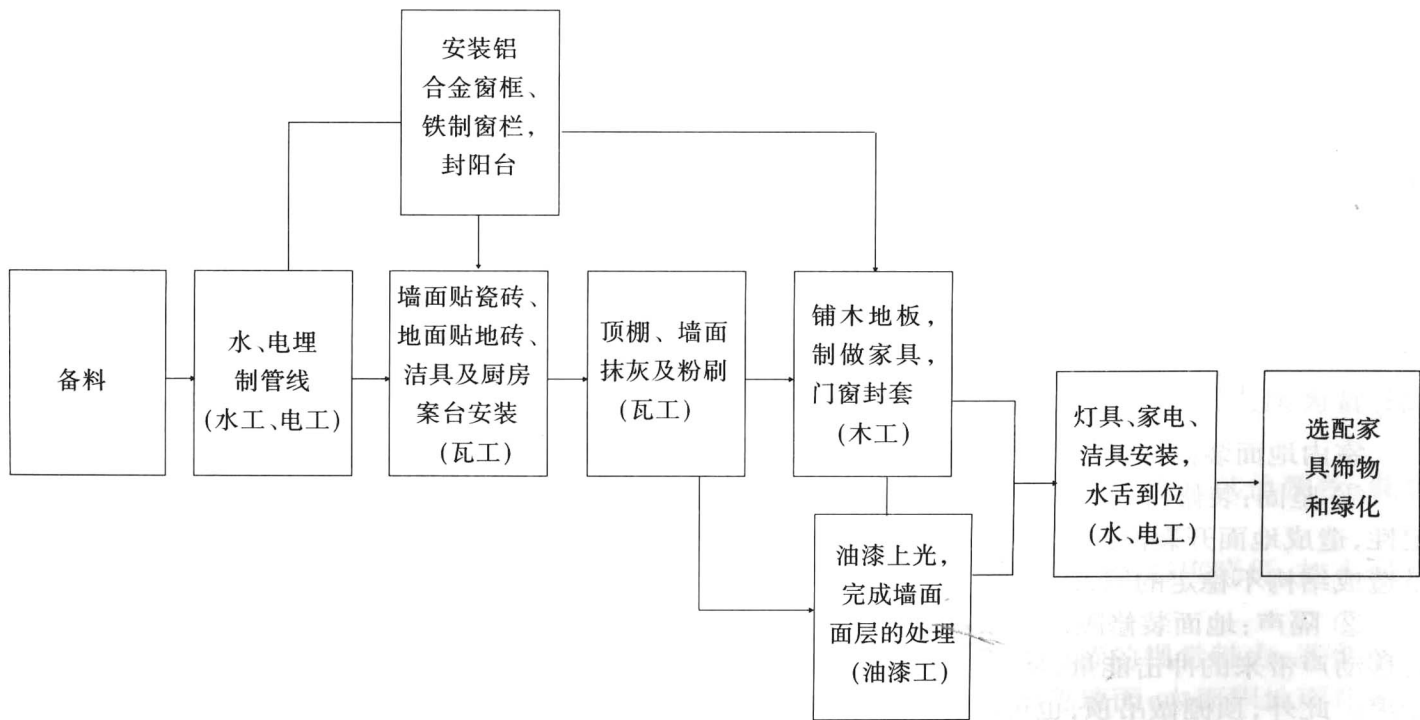
图 1 家庭装修工序流程
