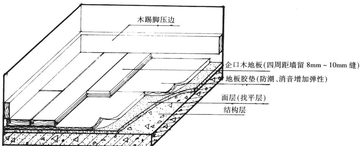
图 12 免漆免刨木地板(快装)构造图
