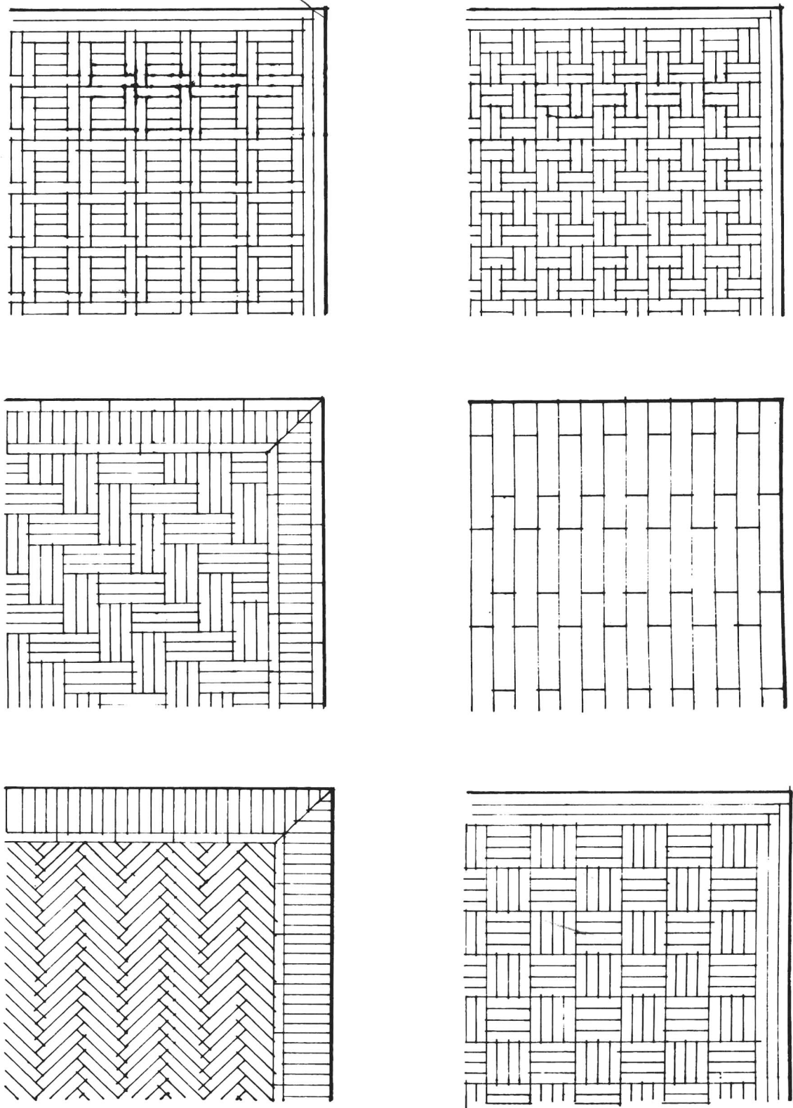
图8 拼花木地板图案举例
