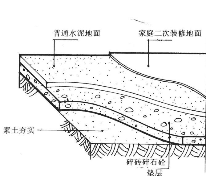
图2 地层地面构造图
