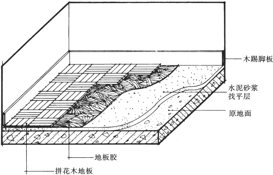
图 7 粘贴式拼花木地板构造图
