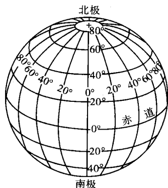
图 1.8 经纬网
