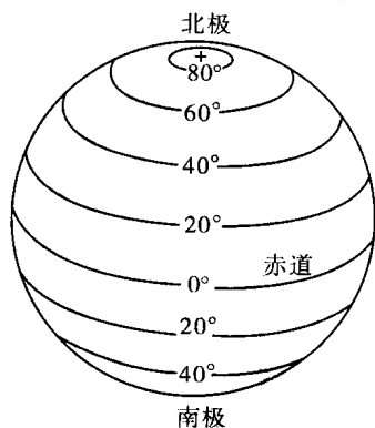
图 1.4 纬线和纬度
