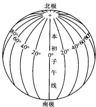
图 1.6 经线和经度
