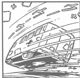
救护车声
