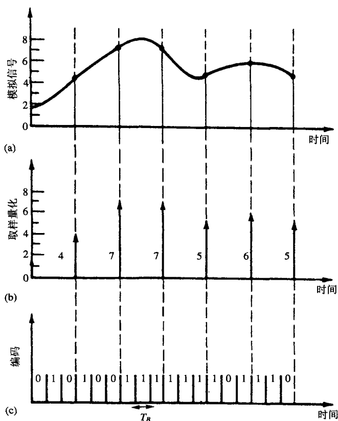
图 1.5 模拟信号转变成数字信号
