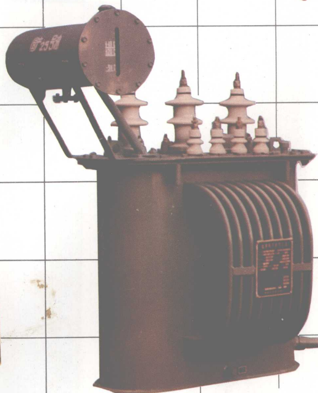
SP-250/10 低消耗節能變壓器
