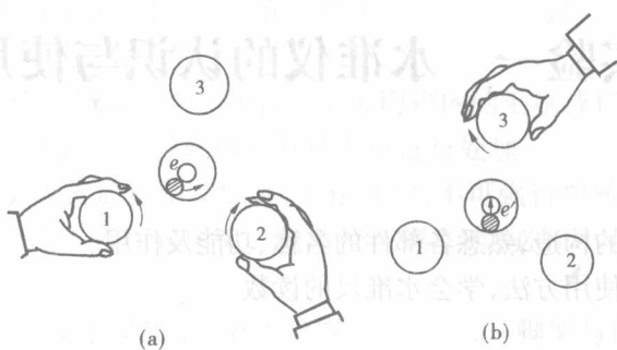
实验图1 概略整平方法
