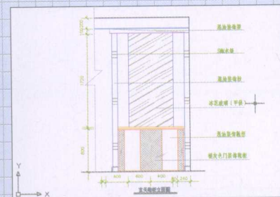
一室一厅一卫户型玄关鞋柜立面图
