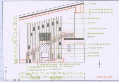
跃层式户型电视主墙立面图
