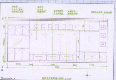
两室两厅一卫户型客厅立面图
