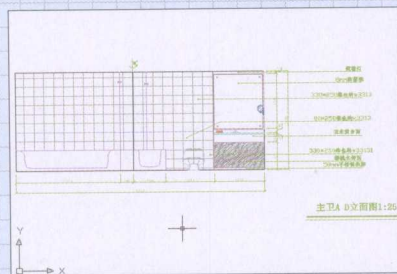
三室两厅两卫户型主卫立面图
