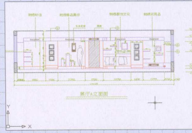
展示厅立面图
