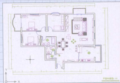
三室两厅两卫户型平面布置图
