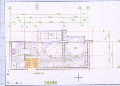
一室一厅一卫(带阳台)户型平面布置图
