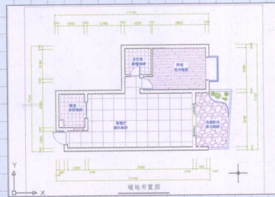
一室一厅一卫户型铺地布置图
