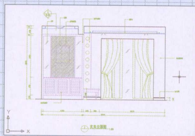
一室一厅一卫(带阳台)户型玄关立面图
