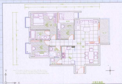
四室两厅两卫户型平面布置图
