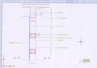
两室一厅一卫户型餐厅墙面剖面图
