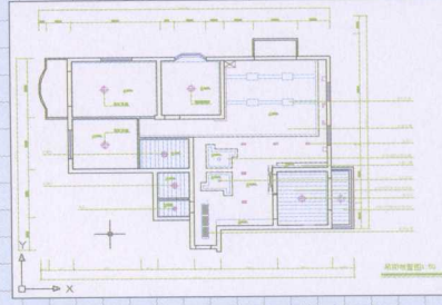
三室两厅两卫户型天花布置图
