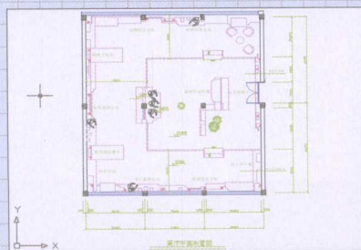
展示厅平面布置图
