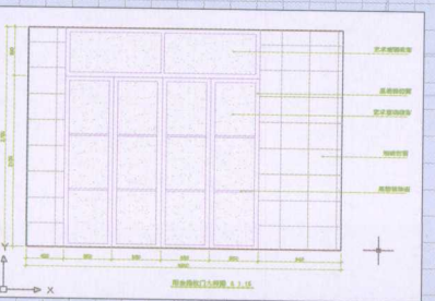
两室两厅一卫户型阳台推拉门大样图
