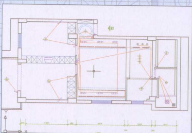
两室两厅一卫户型开关布置图
