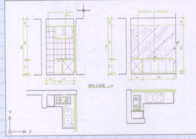
一室一厅一卫户型厨房立面
