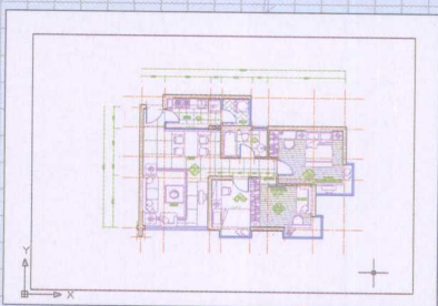
两室一厅一卫户型平面布置图
