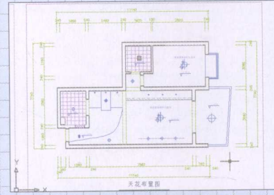
一室一厅一卫户型天花布置图
