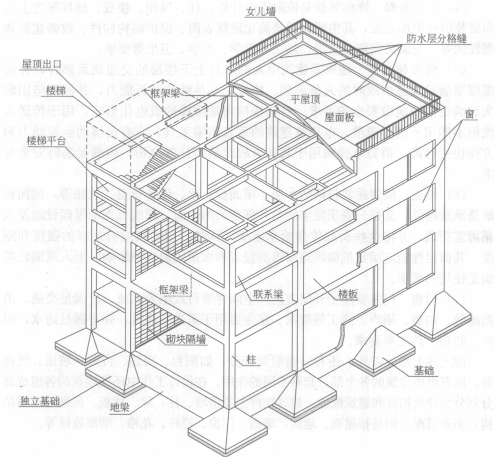
图 1-2 钢筋混凝土框架结构的建筑构造组成
