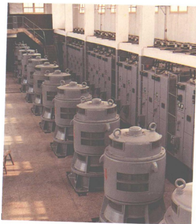
滁河红山窑翻水站机泵房
