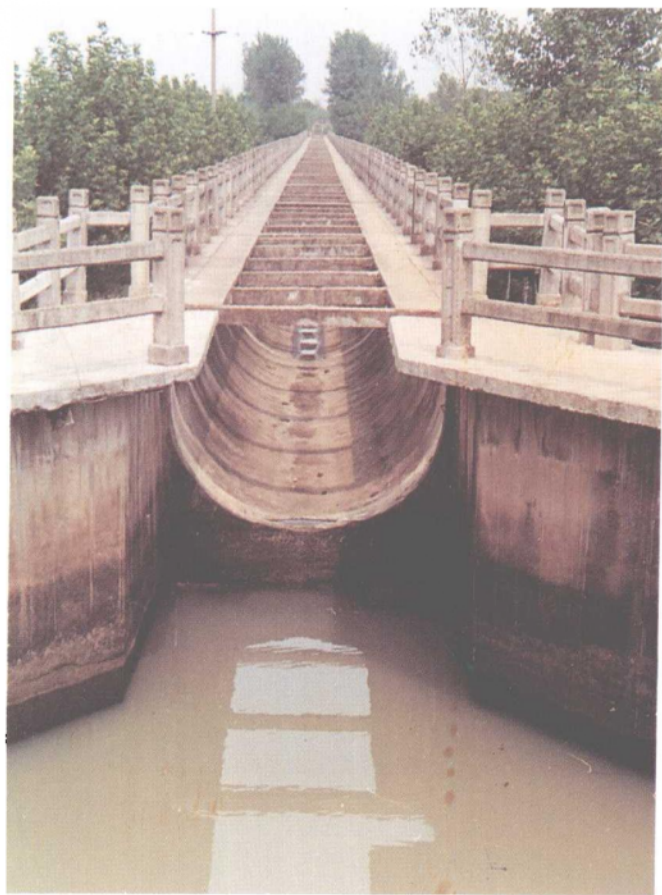
引彌補庫U型薄壳渡槽
