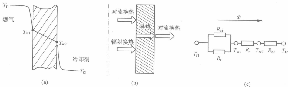
图 1-3 传热过程剖析
