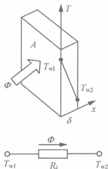
图 1-1 通过平壁的导热
