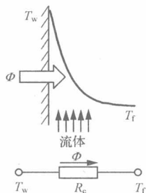
图 1-2 对流换热
