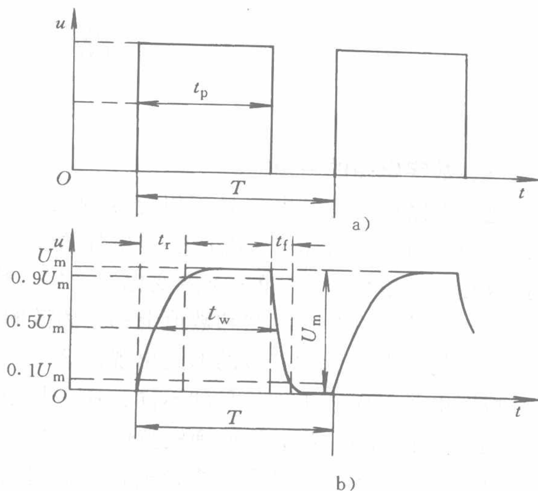
图 0-2 矩形电压的参数
