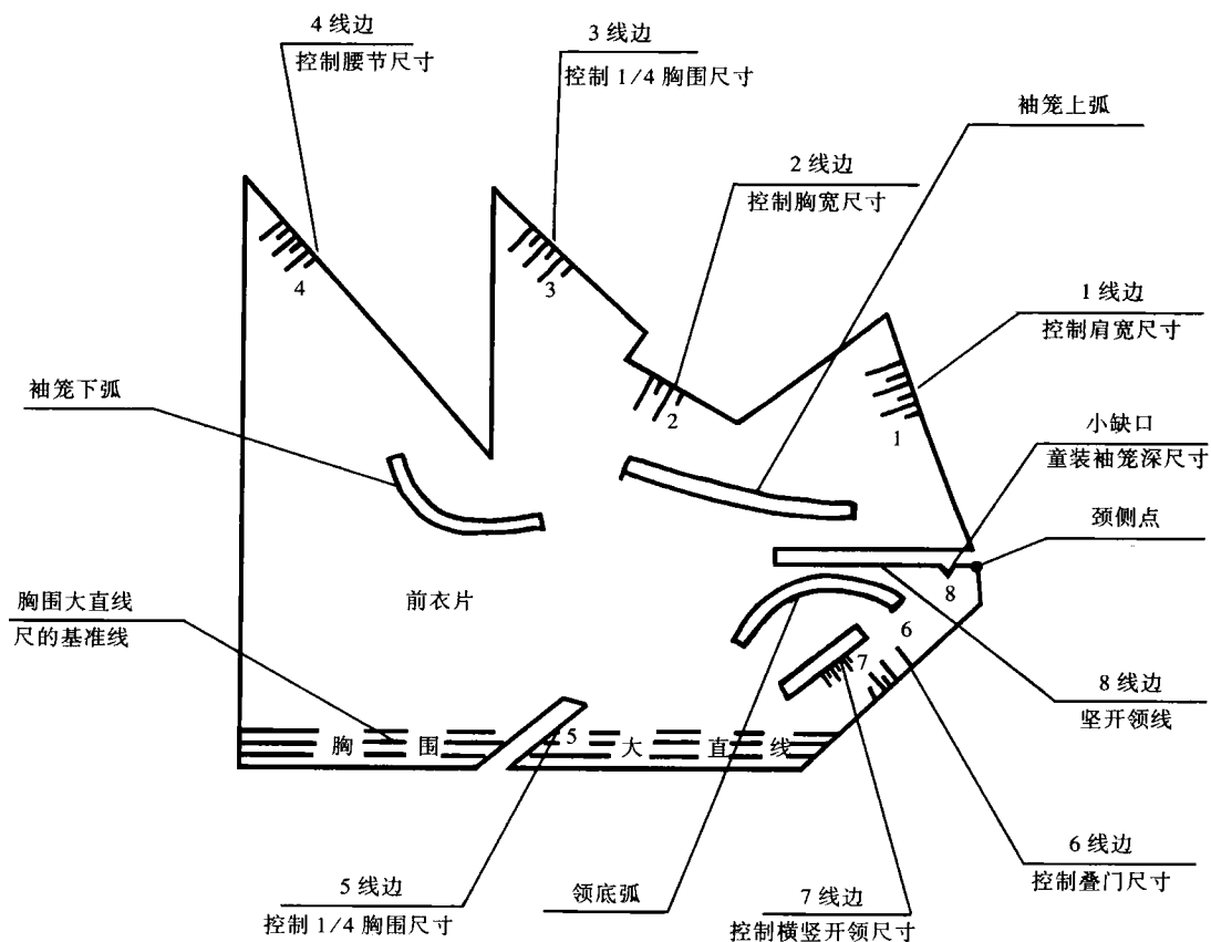
图 1.1 傻瓜裁剪前衣片尺
