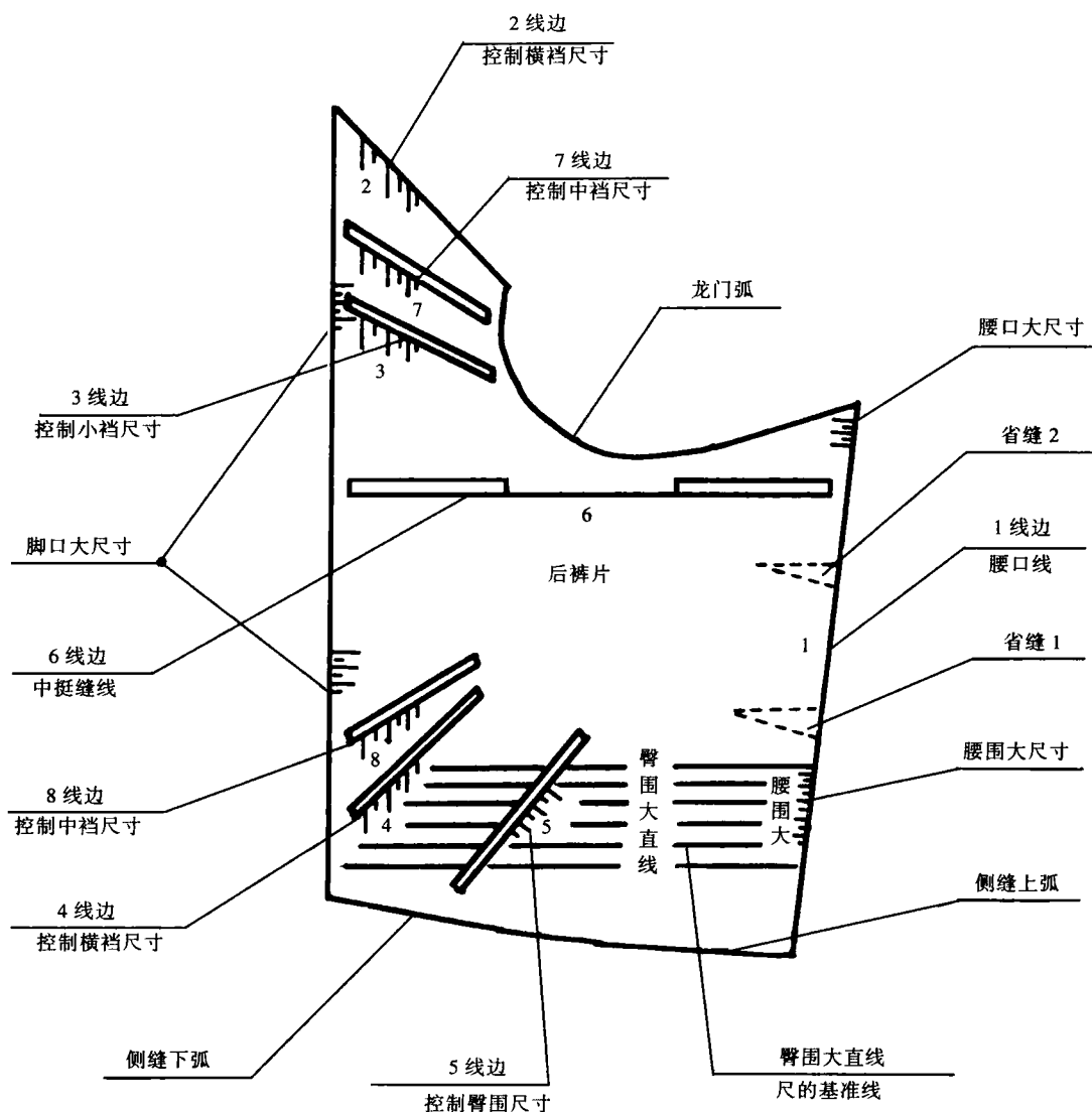
图 1.5 傻瓜裁剪后裤片尺
