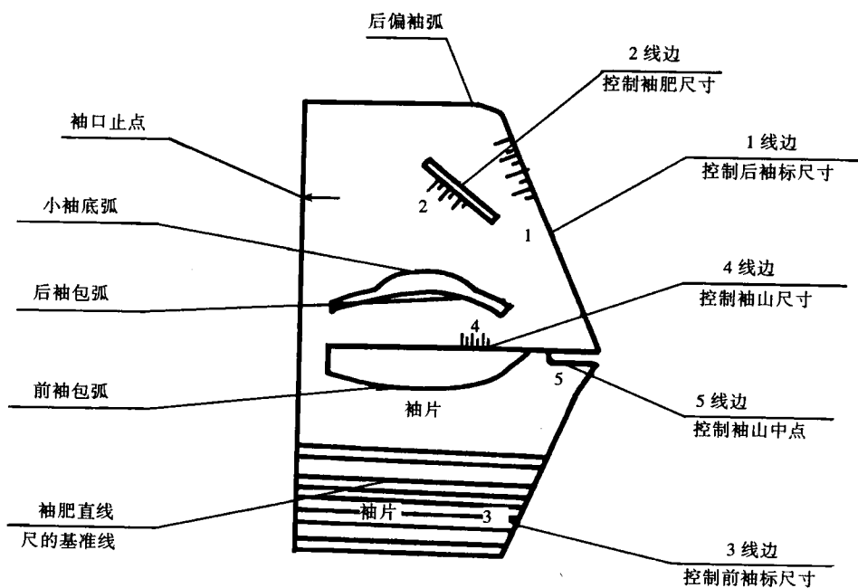
图 1.3 傻瓜裁剪袖片尺
