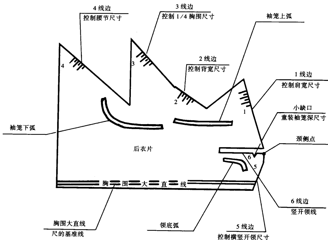
图 1.2 傻瓜裁剪后衣片尺
