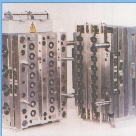
▲ 高精度的熱流道注塑模具
