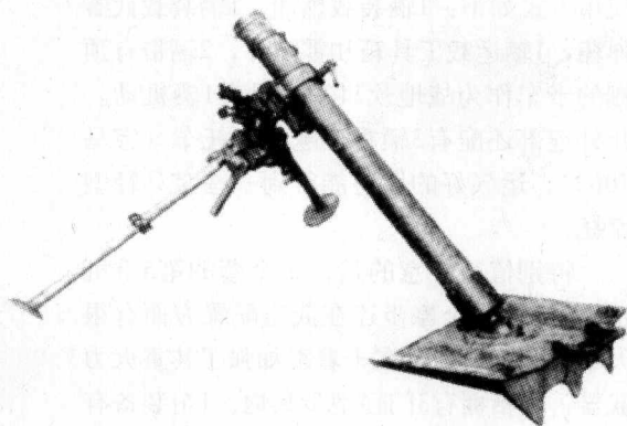
80毫米GrW34中型迫击炮侧后视图
