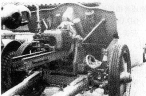
从不同角度拍摄的I. FH. 18型105毫米榴弹炮
