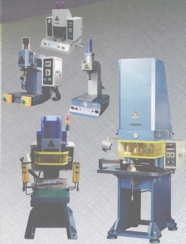
气液增压型气动压力机系列，多工位气动压力机
