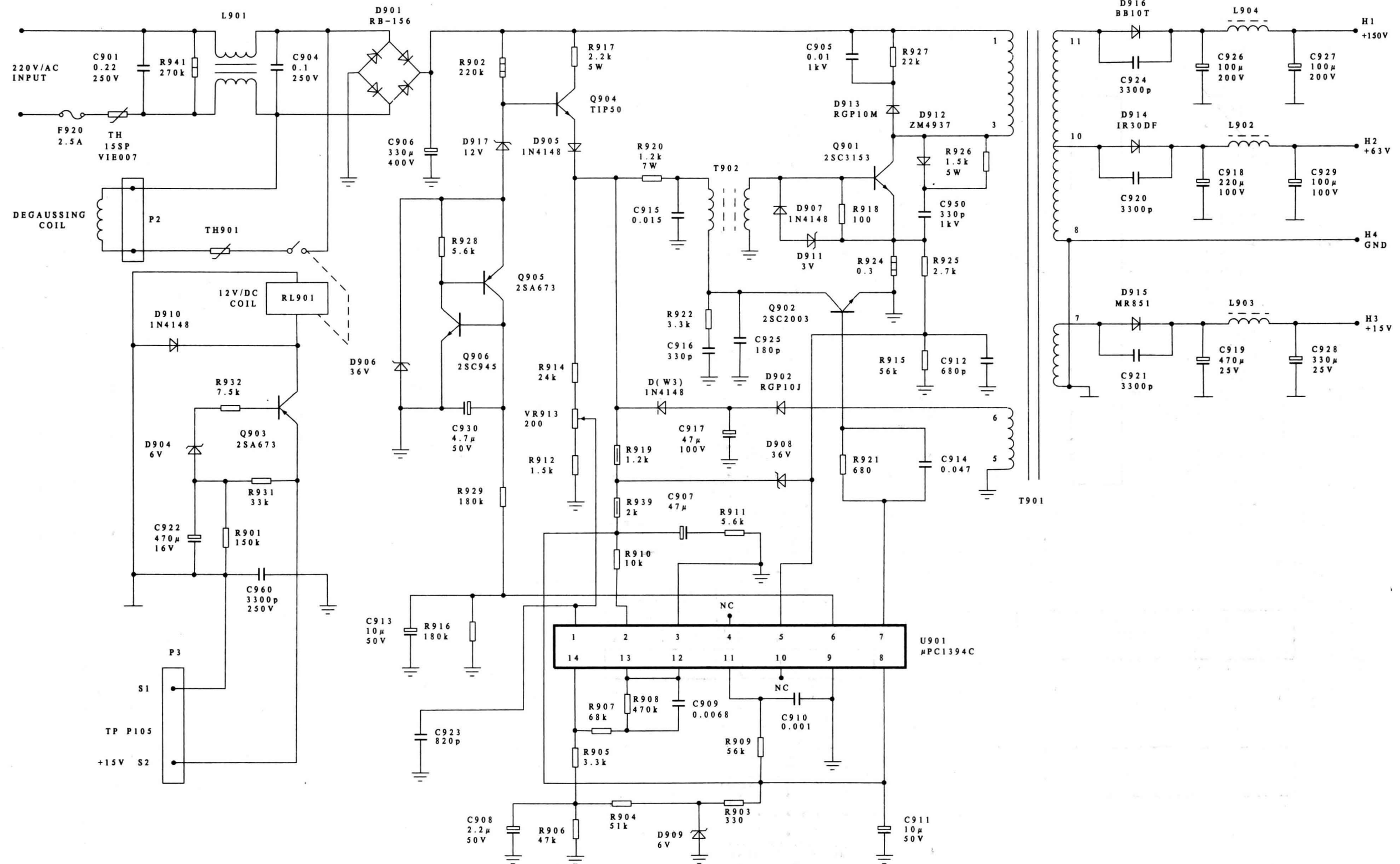
AST ASTECDI彩色显示器电源部分电路图
