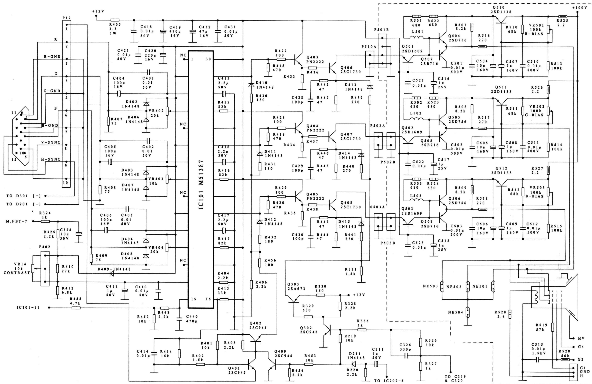
COMPAQ 420型彩色显示器视频处理及放大部分电路图
