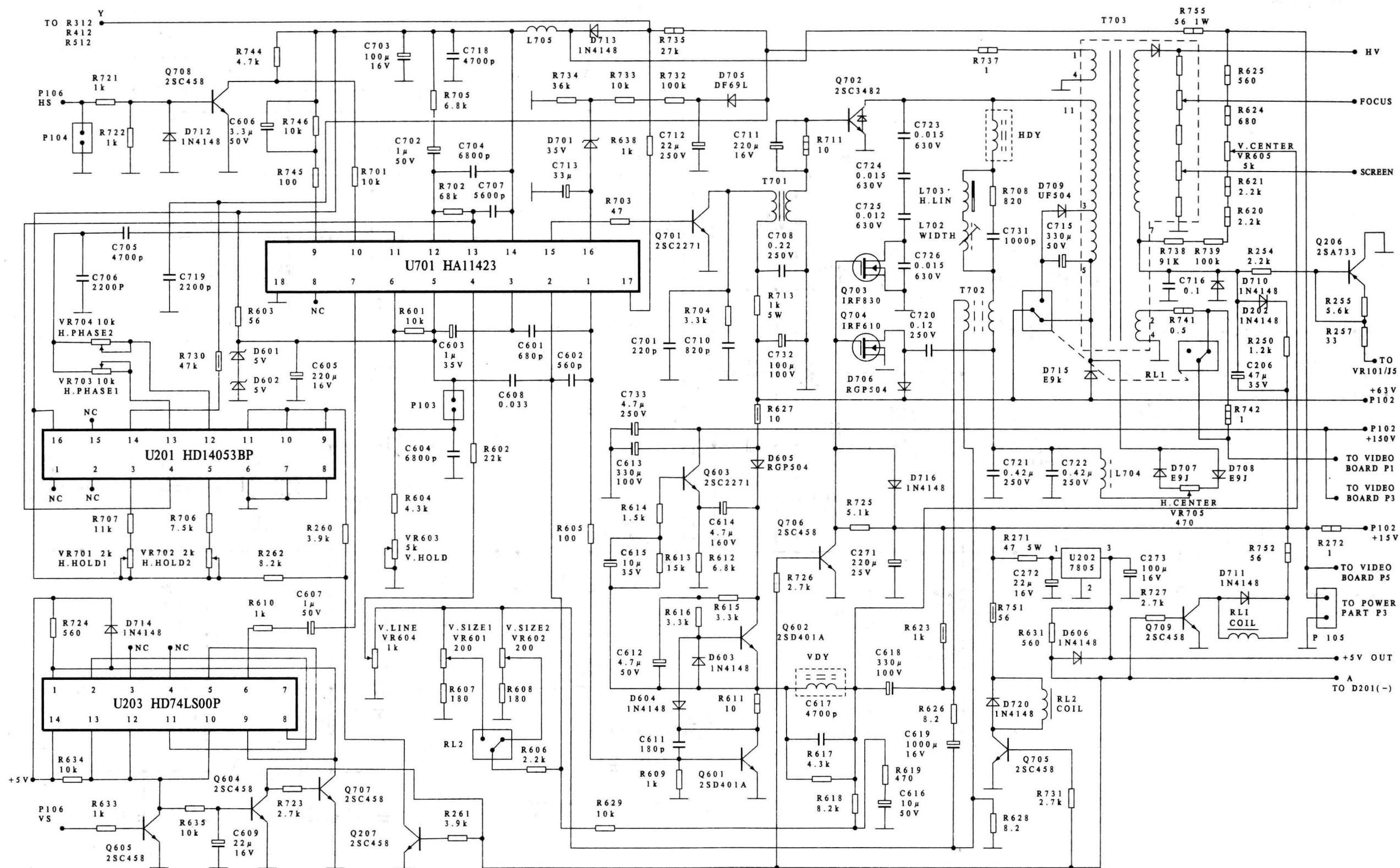
AST ASTEC DI彩色显示器行场扫描部分电路图
