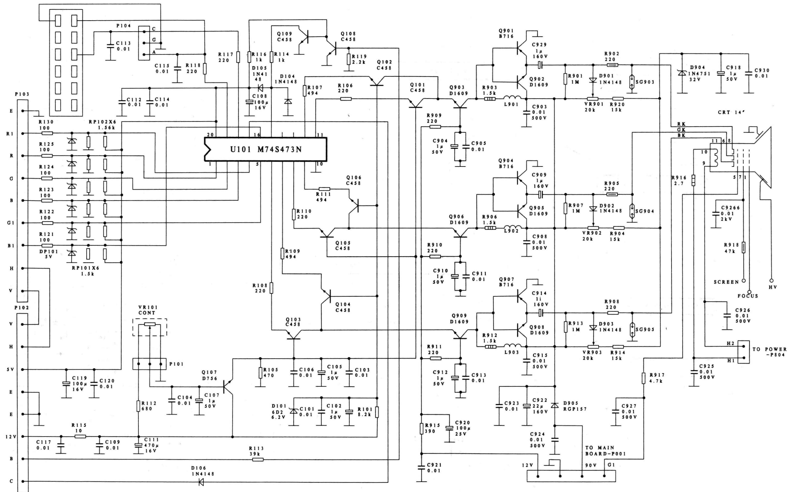
CASPER TM-5154Y型彩色显示器视频输出部分电路图
