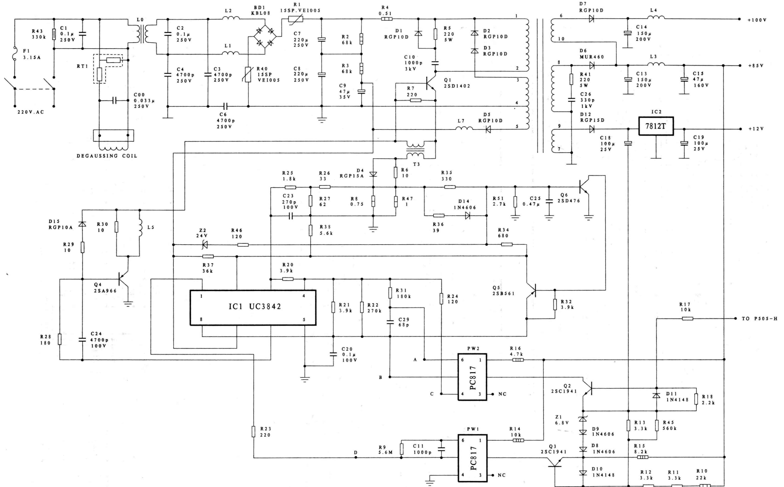
COMPAQ 420型彩色显示器电源部分电路图
