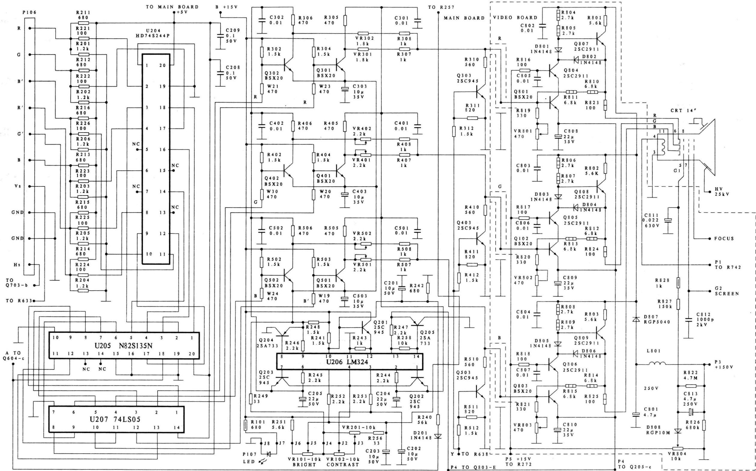
AST ASTEC DI彩色显示器视频处理及放大部分电路图
