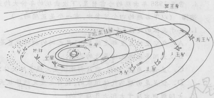
太阳系的模式
