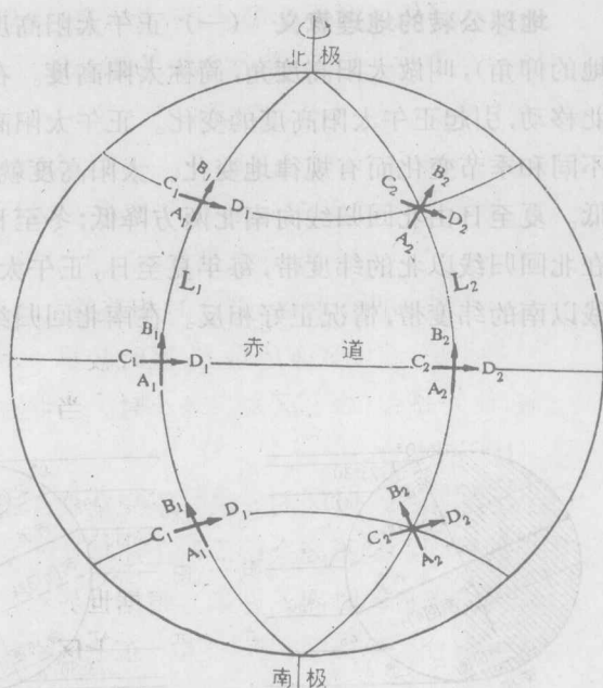
运动物体的水平偏向(赤道上无偏向)
