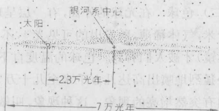
银河系示意(侧视)
