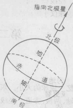
地轴、两极和赤道
