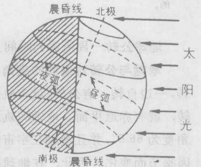
昼半球和夜半球
