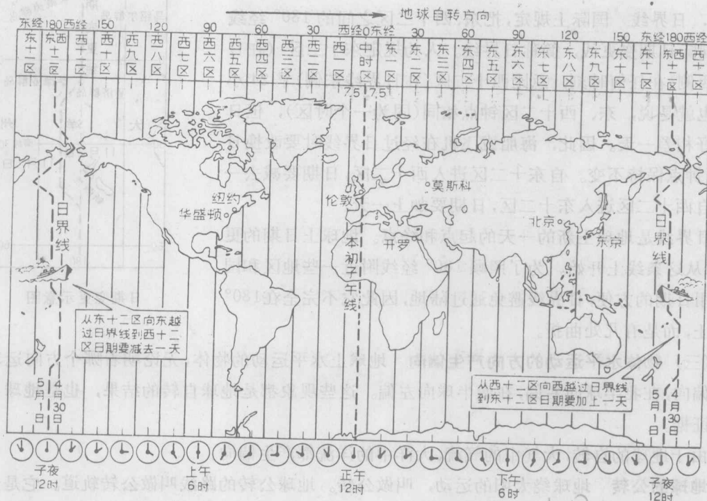
时区和日界线图
