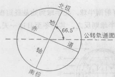
地轴与公转轨道面的夹角
