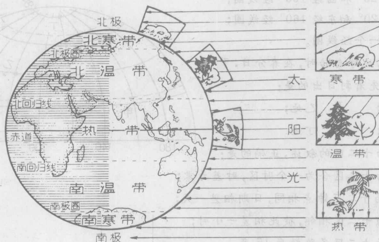
地球上的五带
