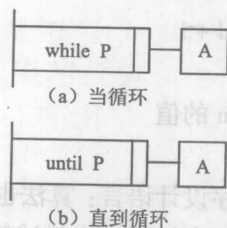
图 1-8 PAD 的循环结构
