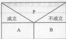
图 1-3 N-S 图的选择结构
