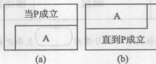
图 1-4 N-S 图的循环结构
