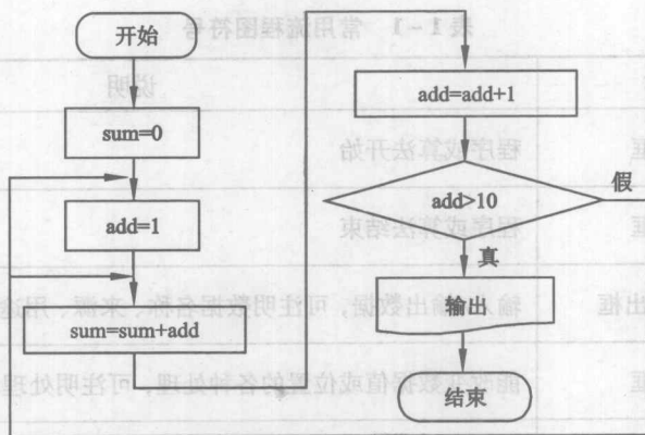
图 1-1 算法 1.1.2 的流程图
