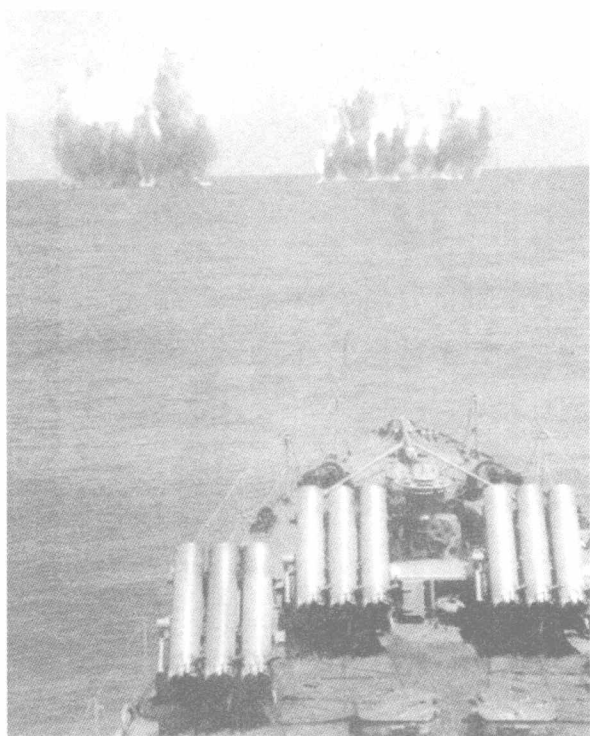
中国猎潜艇发射深水炸弹
