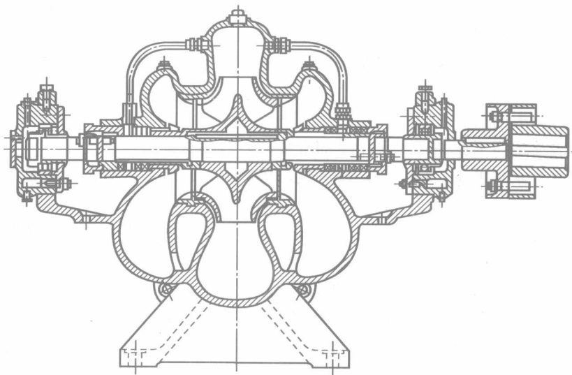
图 1-2 双吸离心泵的结构
