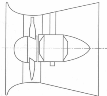
图 1-6 轴流风机的结构
