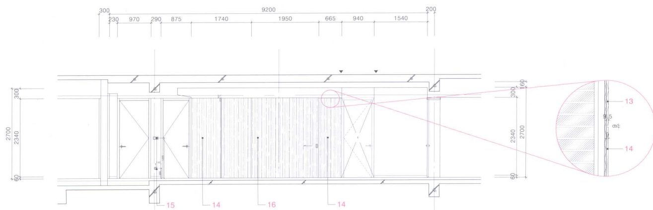
2层起居室立面图 D
