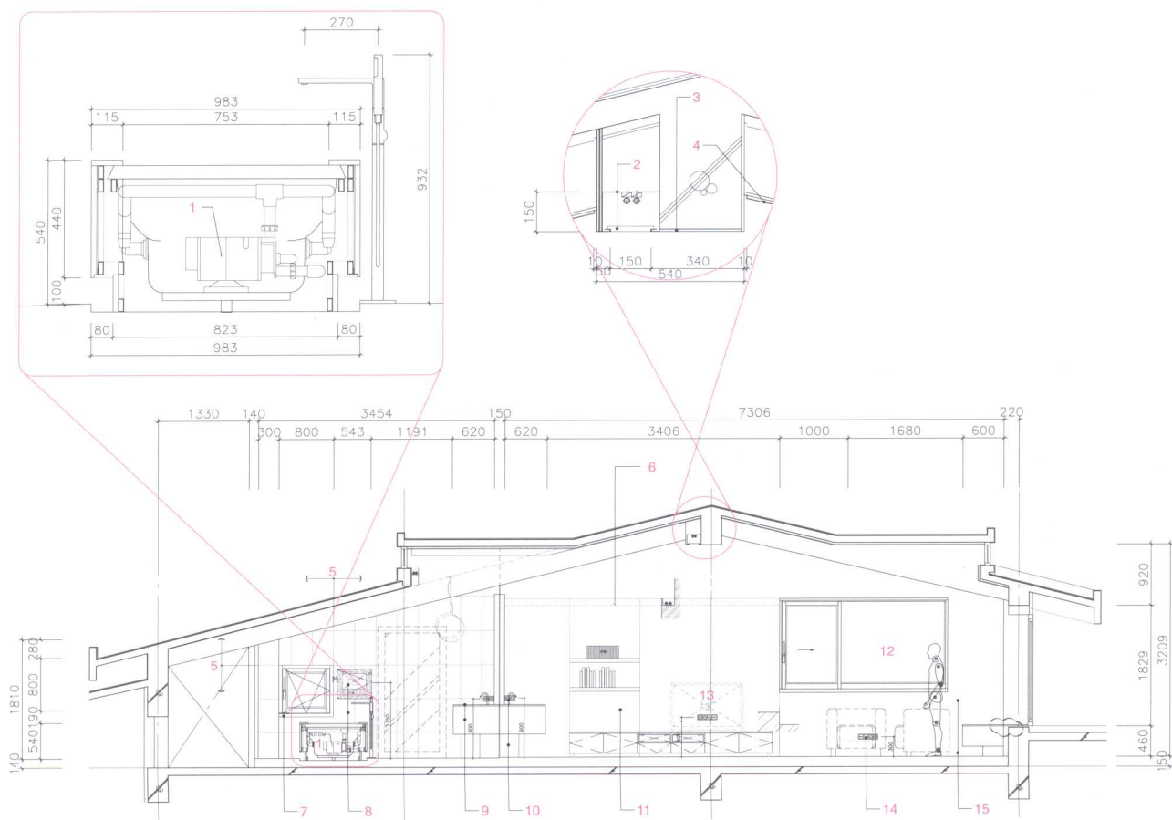
3层主卧立面图O
