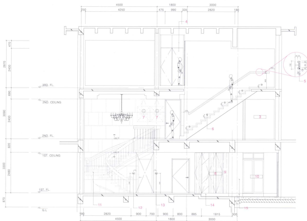
走廊局部剖面图M
