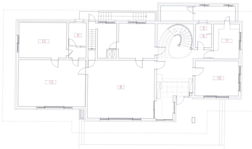
1 层平面图
