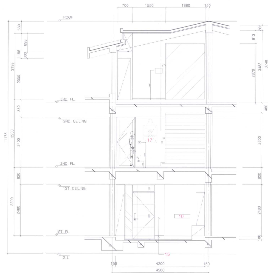
走廊局部剖面图N
