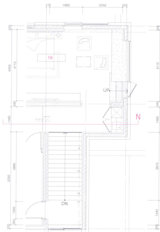
3层走廊局部地板平面图
