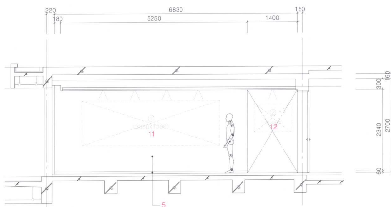
2层起居室立面图 A
