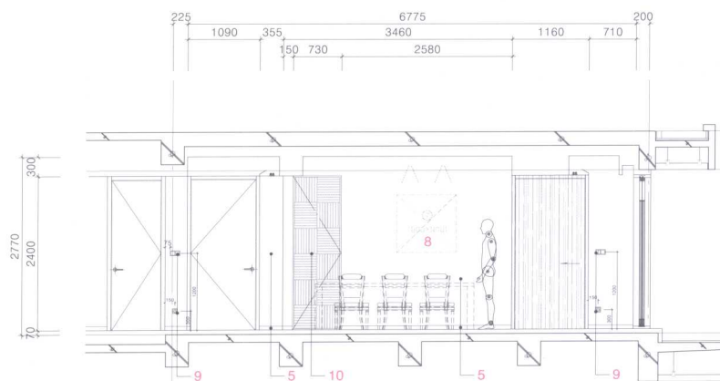
2层起居室立面图 C
