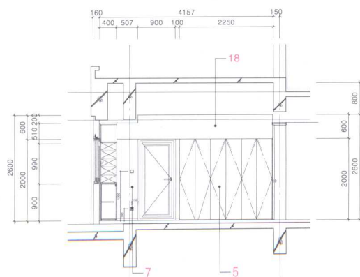
2层B型房立面图K
