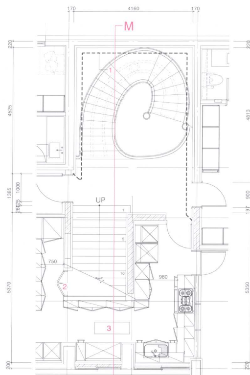
2层走廊局部平面图
