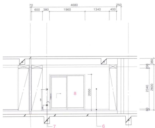
2层A型房立面图G
