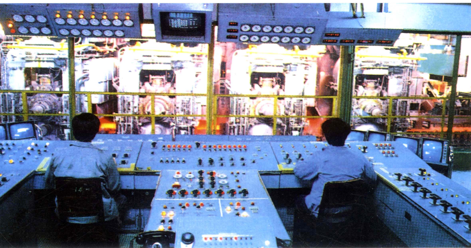
武汉钢铁（集团）公司“一米七”精轧机控制室
