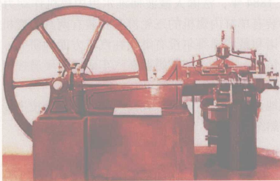
图1-24 奥托制成的卧式四冲程煤气内燃机
