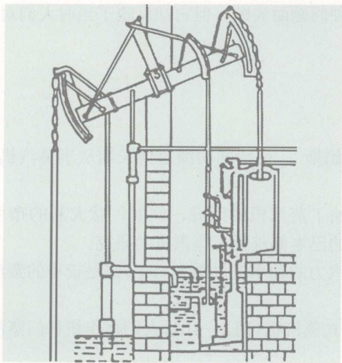
图 1-12 瓦特的第一台蒸汽机
