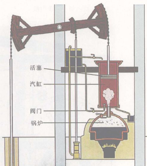
图1-10 纽科门蒸汽机
