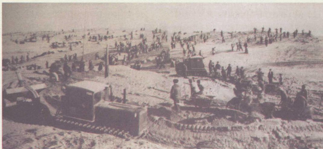
1959年11月西干渠工程建设工地
