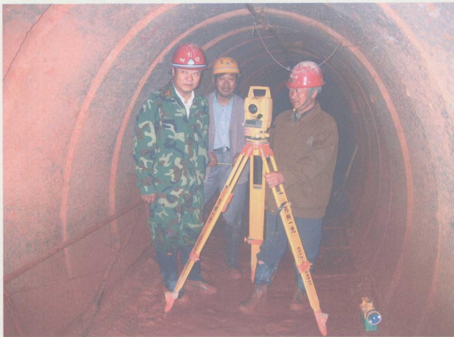
六盘山引水工程牛营隧洞施工
